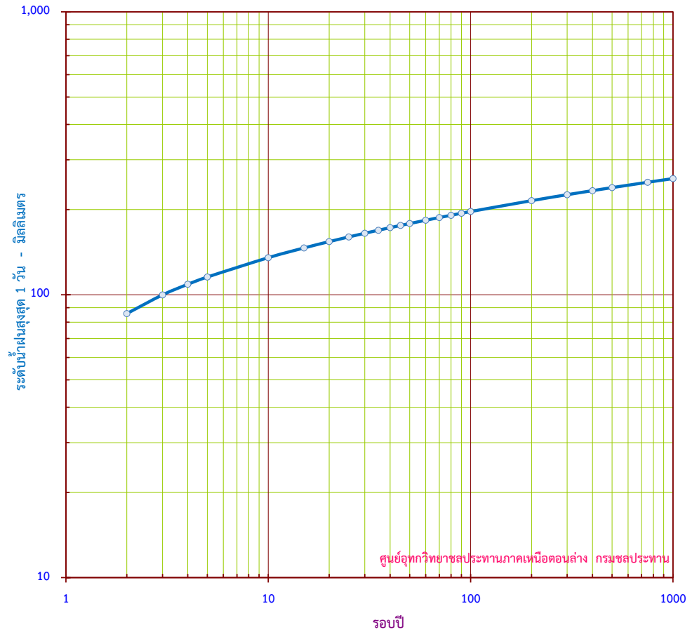
กราฟแสดง ปริมาณน้ำฝนสูงสุด1วัน ขนาดรอบปีต่างๆ สถานี 700221 อ.ตรอน จ.อุตรดิตถ์
